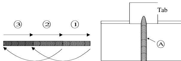
Fig. 6.8 a. Step back technique
