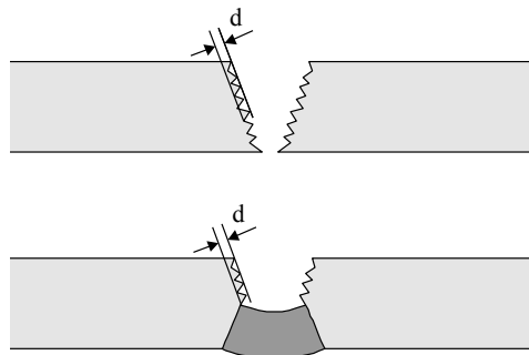
Fig. 6.1. Groove roughness
